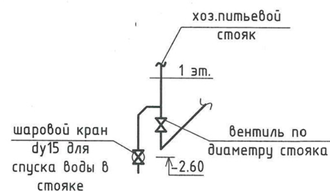
Узел установки спускных кранов на стояках холодного и горячего хоз.питьевого водоснабжения.
